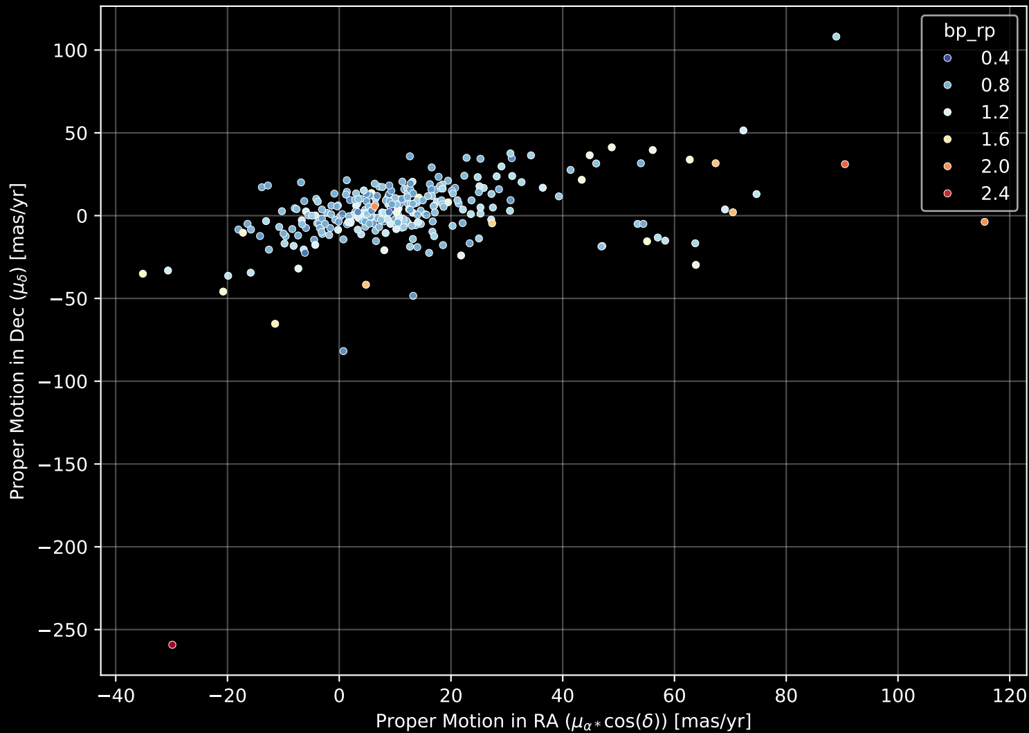
GALAH DR4 Field: [6920] Proper Motion Diagram (n= 300)
