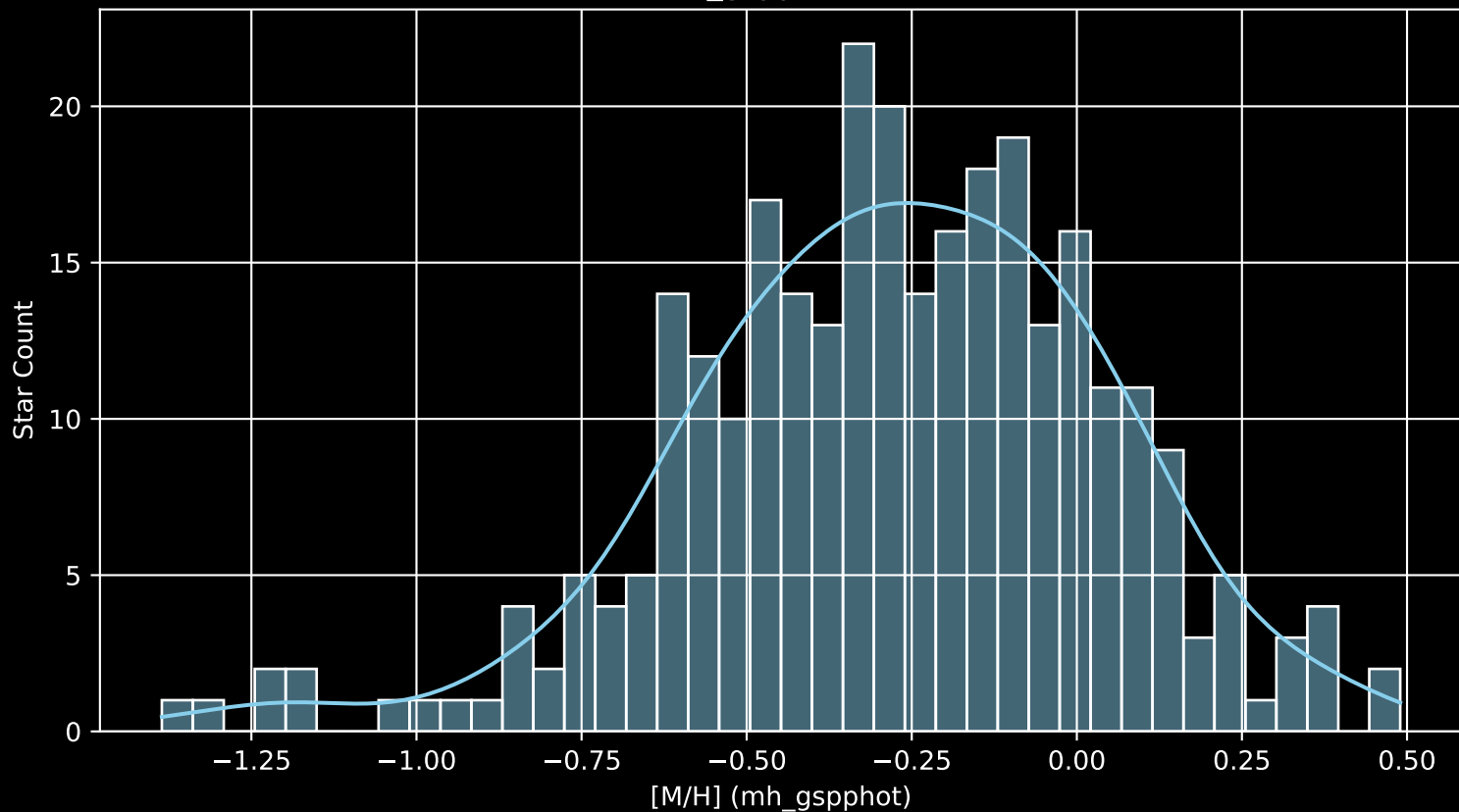
GALAH DR4 Field: [6920] [M/H] (mh_gspphot) (n= 297)
