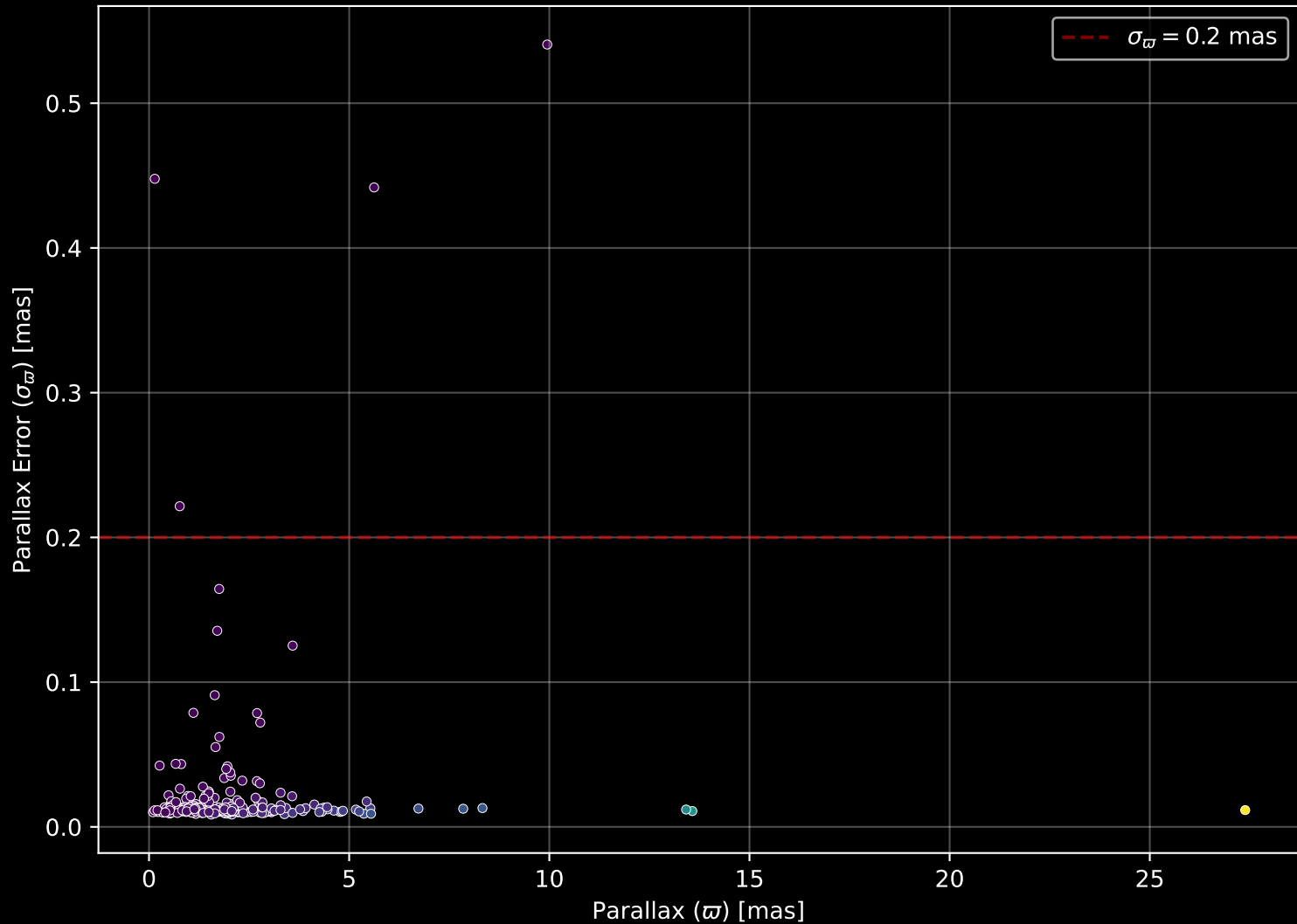
GALAH DR4 Field: [6920] Parallax Quality (n= 300)
