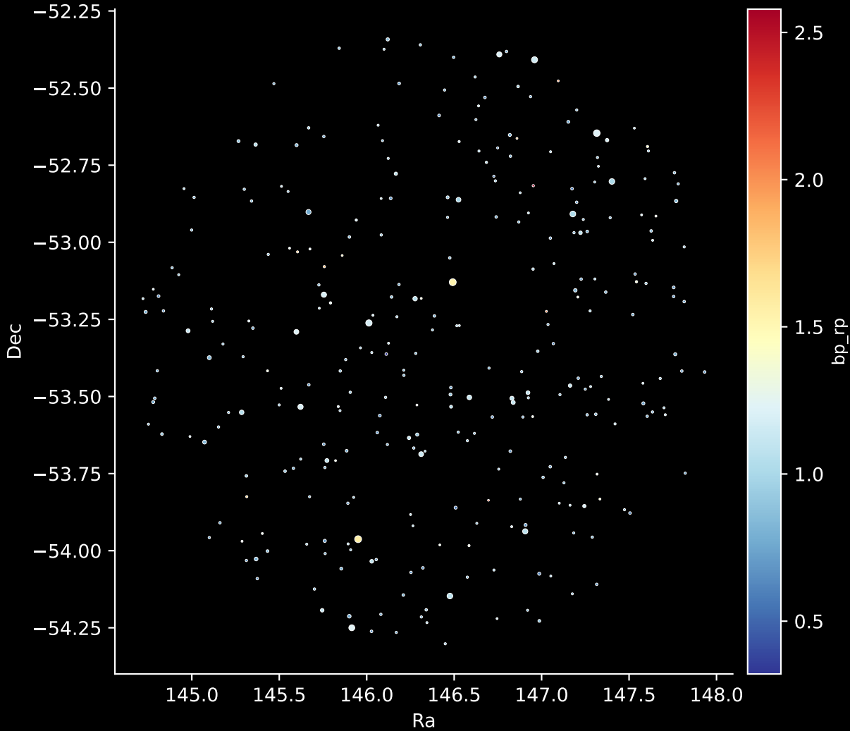
GALAH DR4 Field: [6920] Stars: 300
