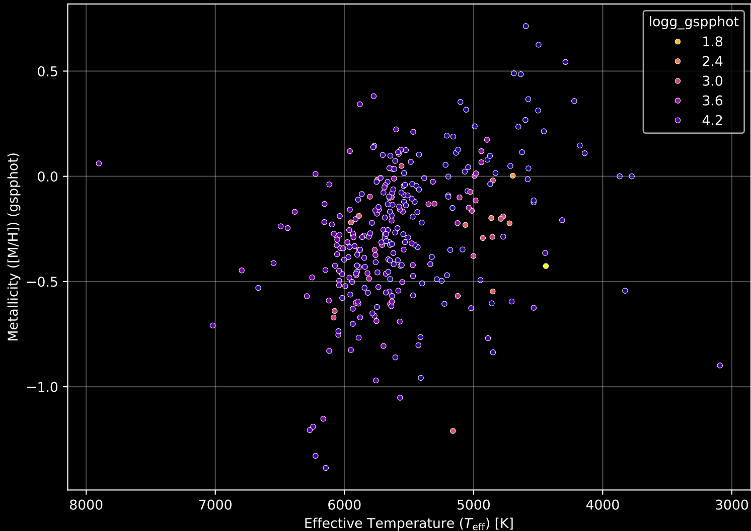
GALAH DR4 Field: [6920] Stellar Population Parameters (n= 300)
